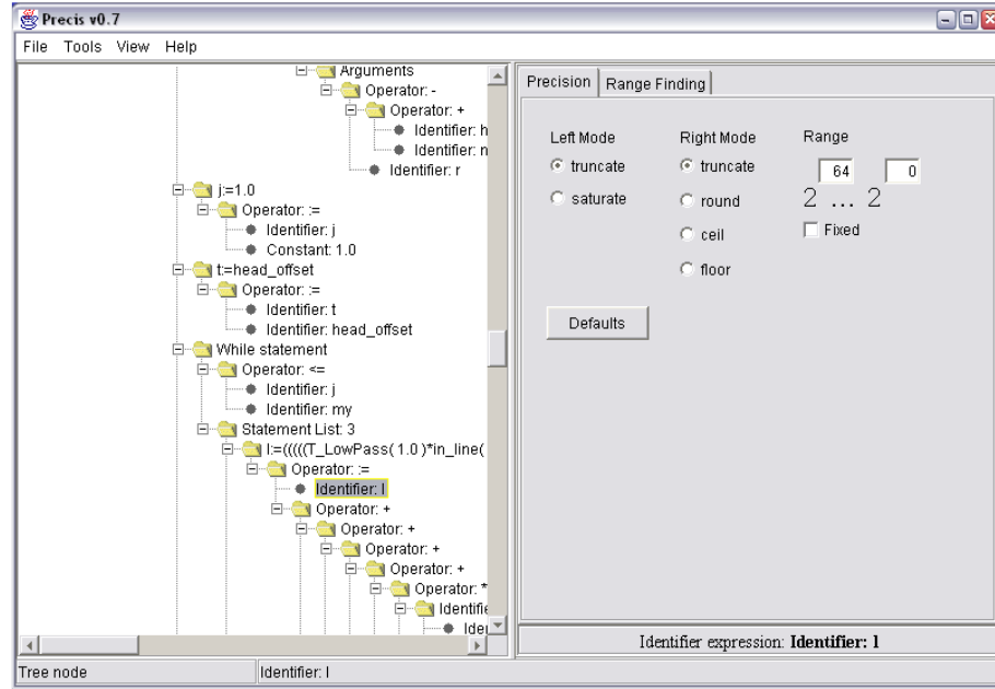
Figure 4.1: Précis screenshot
